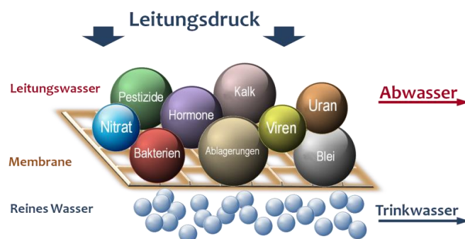
Abbildung: Modell zur Umkehrosmose
